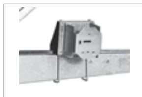
Support roue de secours
