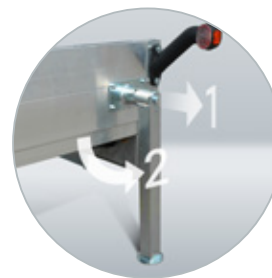
Béquilles faciles à positionner
